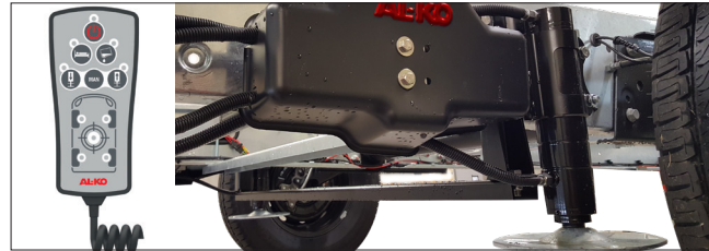
AL-KO HY4 hydraulische Stützen. Justieren Sie Ihr Fahrzeug mit einem einzigen Knopfdruck auf der Fernsteuerung. Mit einem weiteren Knopfdruck richten Sie es bei kleinem Gefälle aus. Das HY4-System kann auch vollständig manuell gefahren werden, indem Sie die verschiedenen Stützbeine individuell steuern. Jede einzelne Stütze hat einen eigenen Antrieb. Das gesamte System wird am Fahrwerk montiert, so dass keine Ölleitungen durch den Aufbau gezogen werden müssen. HY4 ist beim Imperial serienmäßig, beim Novum, Royal und Crown ist es als Zubehör erhältlich.
