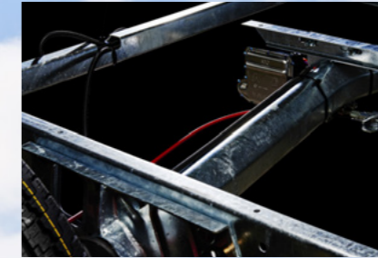
Besonders verdrehsteifes Fahrwerk. Zusätzliche Traversen zwischen den Längsträgern des Fahrwerks verstärken den Fußboden und erhöhen die Verdrehsteifigkeit des Chassis. Die Chassis haben Ausleger von den Längsträgern zur Entlastung der Spannungen zwischen Fußboden und Wand. Die Karosserie ist für sehr hohe Belastungen ausgelegt, beispielsweise für große Schneelasten auf dem Dach.
